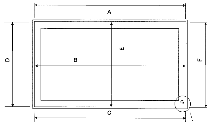
【枠平面図】 ※A~F全て枠の内側を計測
